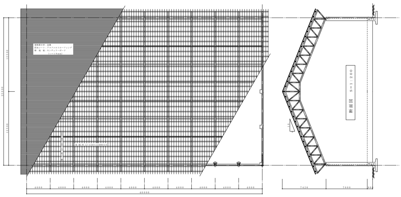
屋根伏図 S=1:200
